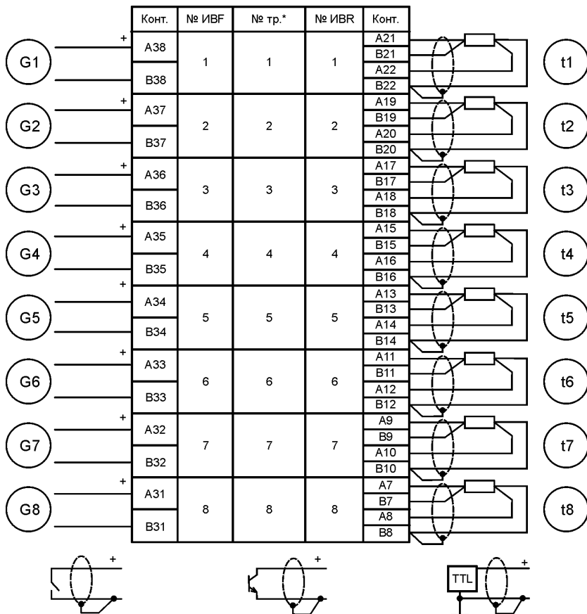
Виды выходных цепей датчиков расхода G1...G8
