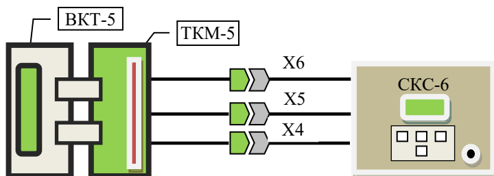
Рис. Б.2 Схема проверки БКТ-5 с использованием СКС-6 и ТКМ-5 Разъемы X4...X6 (ТКМ-5) подключаются к одноименным разъемам стенда СКС6
