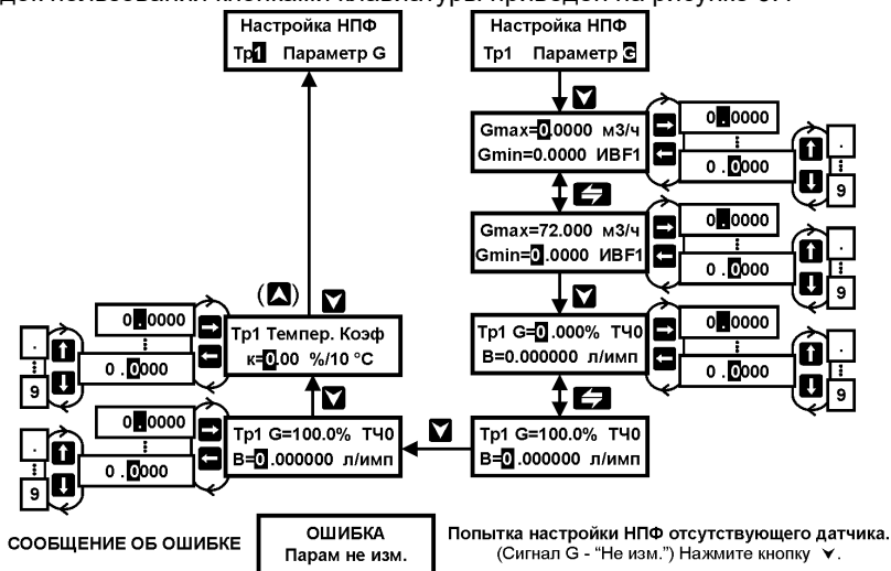
Рисунок 6.4. Настройка НФП для токового и частотного датчиков расхода.
